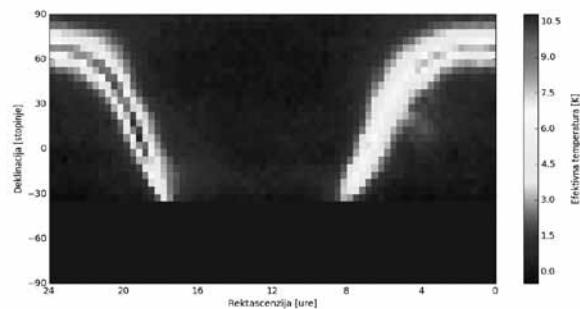
Slika neba z radijskim teleskopom
